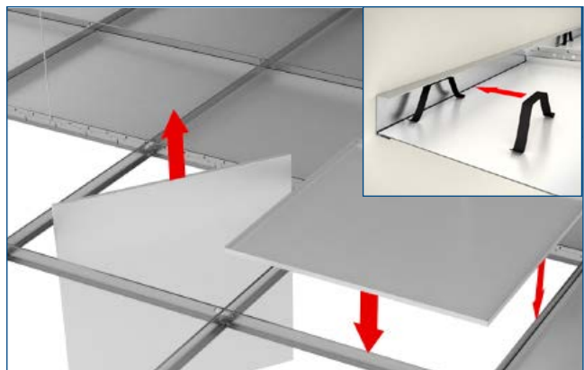
4. Mise en œuvre du plafond
