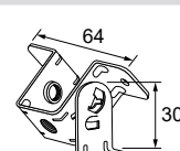
Attache articulée 3D
