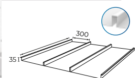
Bacs auto. SG4 à joint creux
