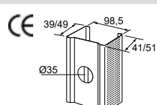
Montants 100
