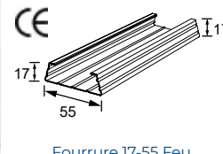
Fourrure 17-55 Feu
