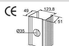
Montants 125
