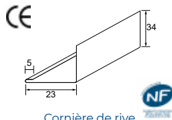
Cornière de rive
