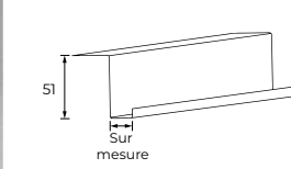
Profil d'accroche
