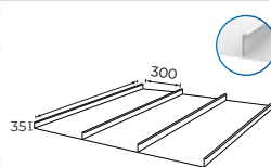
Bacs auto. SG3 recouvrement
