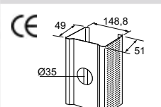
Montants 150
