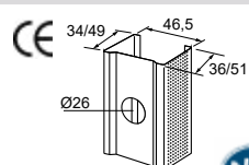
Montants 48
