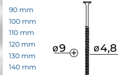
Tête trompette pointe clou
