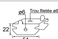
Cavalier 18-45 / 17-47 Milieu humide
