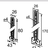
Suspentes NT fourrure 17-47
