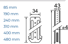
Suspentes fourrure 17-47
