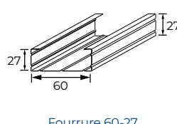
Fourrure 60-27
