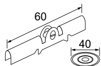
Bascule avec rosace
