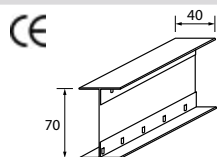
Profil Omnifix 70 - épais. 0,50
