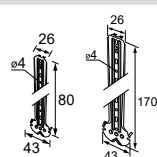
Suspentes NT fourrure 18-45
