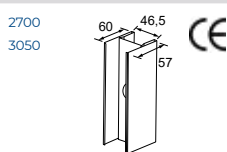
ID + 48
