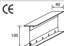
Profil Omnifix 100 - épais. 1
