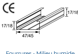
Fourrures - Milieu humide
