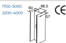
ID + 90 Éclissé
