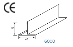
Porteur STI
