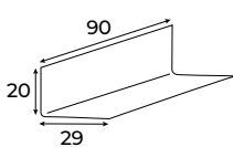
Raccord pour porteur STI
