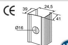
Montants 26
