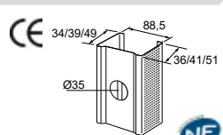
Montants 90
