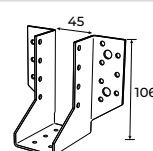
Support pour profil Omnifix
