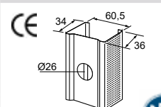
Montants 62
