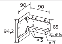
Équerre de fixation Omnifix
