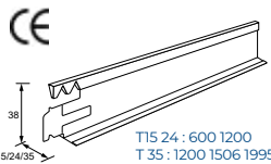
Entretoise
