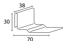
Assemblage taille de pierre
