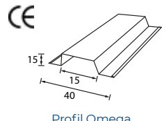
Profil Omega
