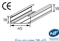
Fourrures 18-45
