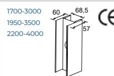
ID + 70 Éclissé
