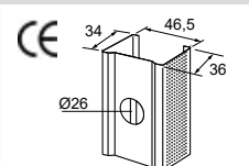
Montants 48 - Milieu humide
