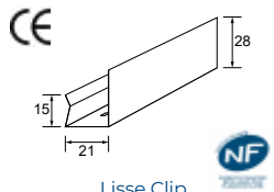
Lisse Clip
