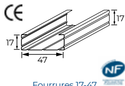
Fourrures 17-47
