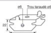
Cavaliers pivot fourrure 18-45 / 17-47
