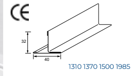
Entretoise STI
