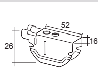
Cavalier droit pour système double scope
