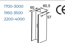
ID + 62 Éclissé
