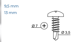
Tête ronde pointe forêt
